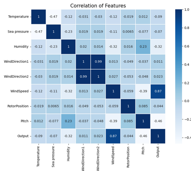
Fig. 3. Data heatmap
